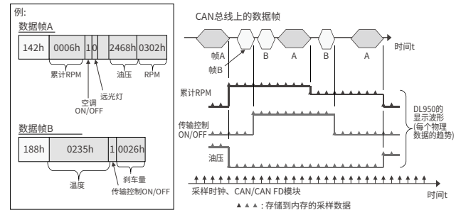
采样数据和显示波形的关系示例
