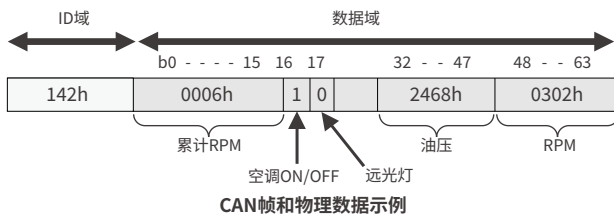
CAN帧和物理数据示例
