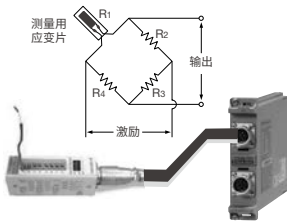
通过应变片测量应变时，通常使用附带的电桥。
